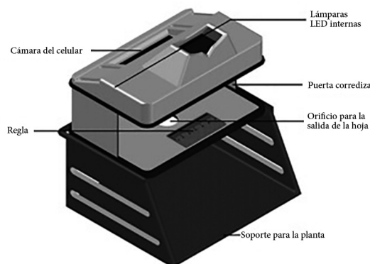
Figura 1. Render del dispositivo empleado para la captura de las imágenes de las hojas de E. crassipes bajo un control de distancia, coplanaridad e intensidad de luz.
